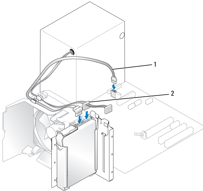
1 직렬 ATA 데이터 케이블 2 전원 케이블
