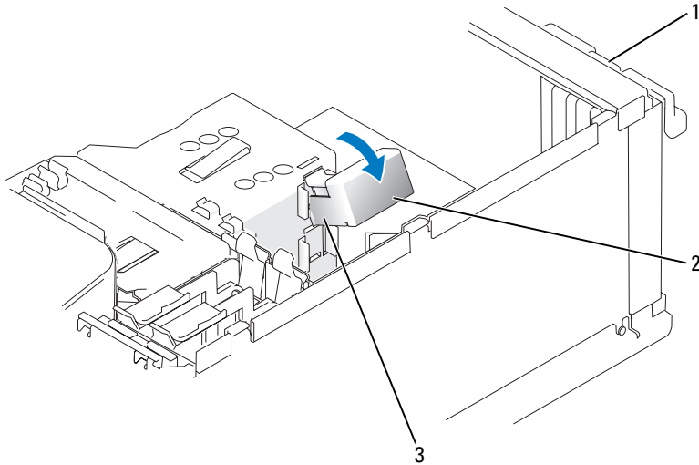
1 카드 고정 도어 2 카드 고정 장치 3 분리 탭 (2 개)
