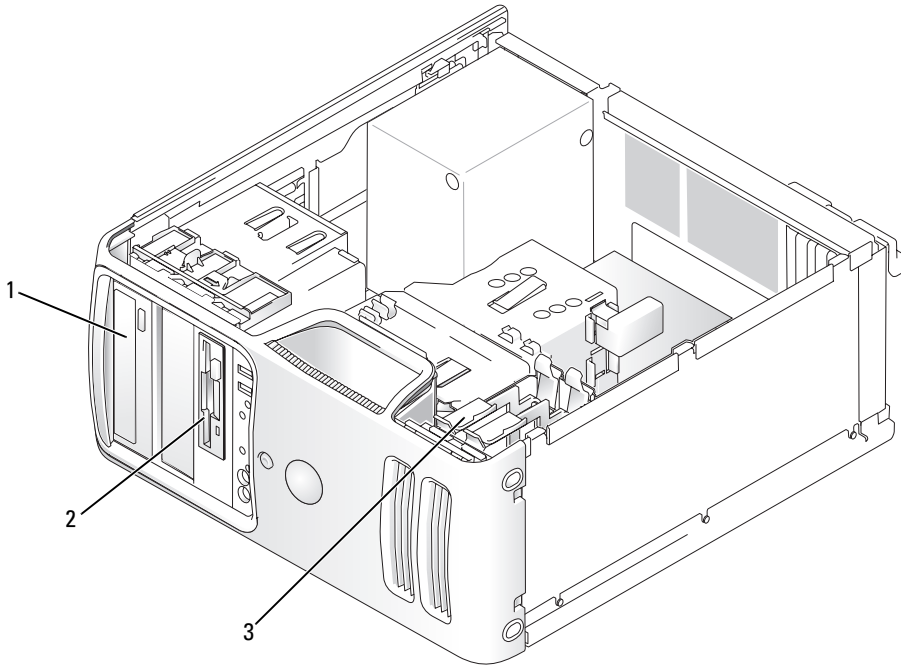
1 CD/DVD 드라이브 2 선택사양인 플로피 드라이브 또는 매체 카드 관독기용 FlexBay 3 하드 드라이브
