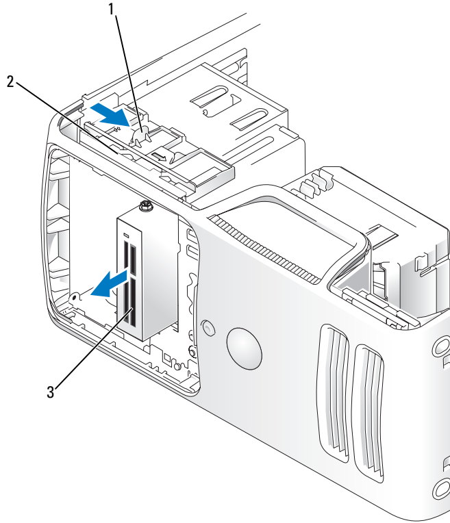
1 드라이브 분리 래치 2 미끄럼판 3 매체 카드 관독기
