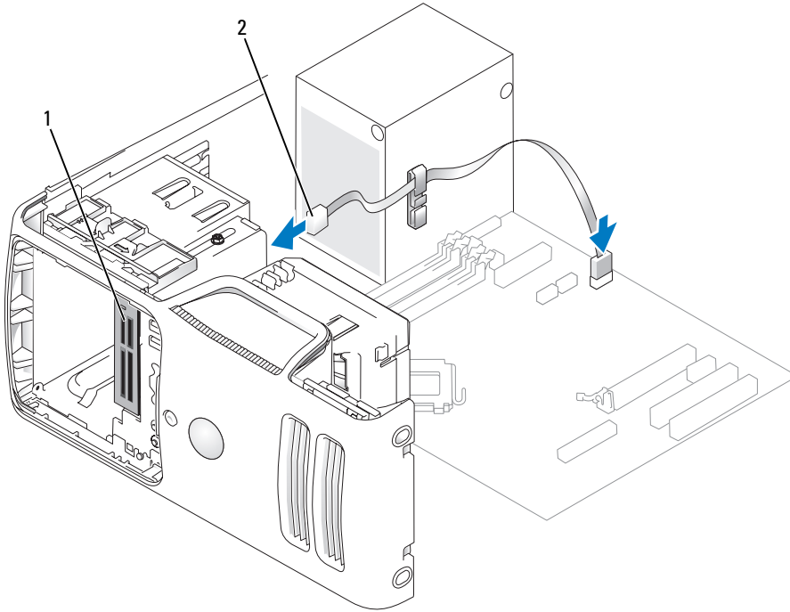
1 매체 카드 관독기 2 FlexBay USB 케이블
